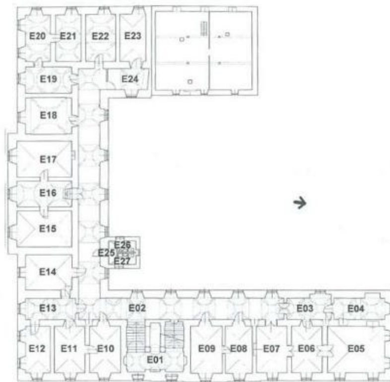
10. kép. Emeleti alaprajz, helyiség számozással. Készült a Litkei Építésziroda Kft. felmérési és átalakítási rajza alapján
