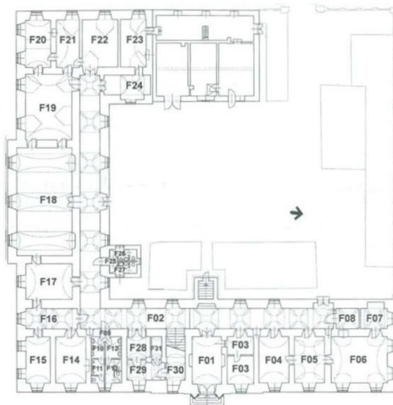
9. kép: Földszinti alaprajz, helyiség számozással. Készült a Látkei Építésziroda Kft. felmérési és átalakítási rajza alapján
