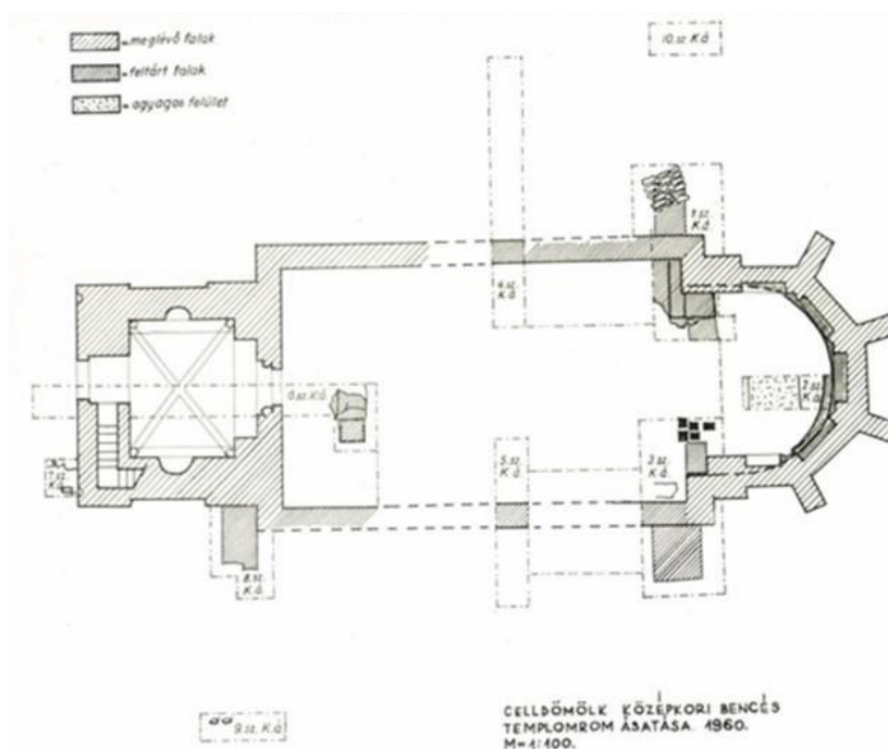
3. kép. A templomrom alaprajza
