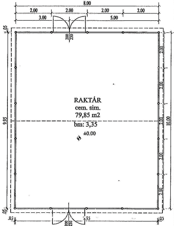
I, J, K, JELŰ RAKTÁR FELMÉRÉSI ALAPRAJZ M 1:100
